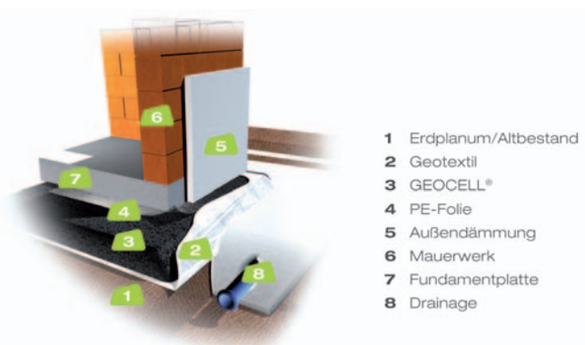
Lastabtragende Dämmung unter der Bodenplatte
